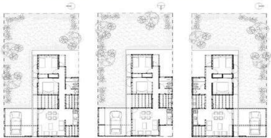
PROTOTIPOS PARA LA ORIENTACIONES RESTANTES
